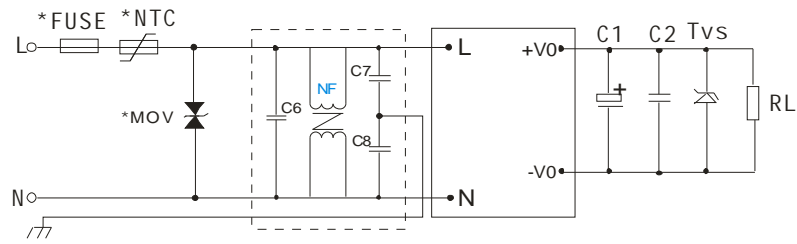
图 3 典型应用电路
