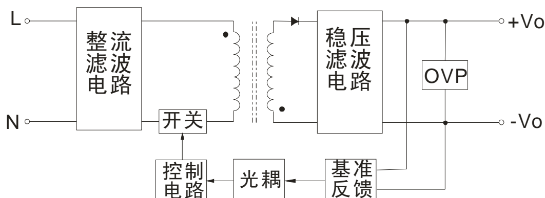
图 1 LD 系列产品原理框图
