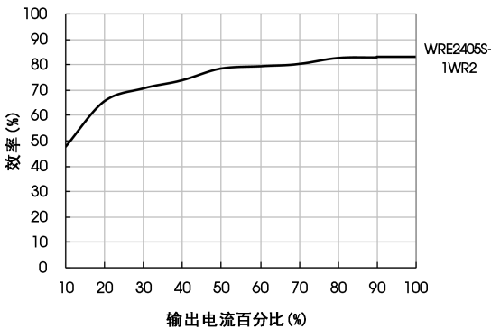
效率Vs输出负载（标称输入）
