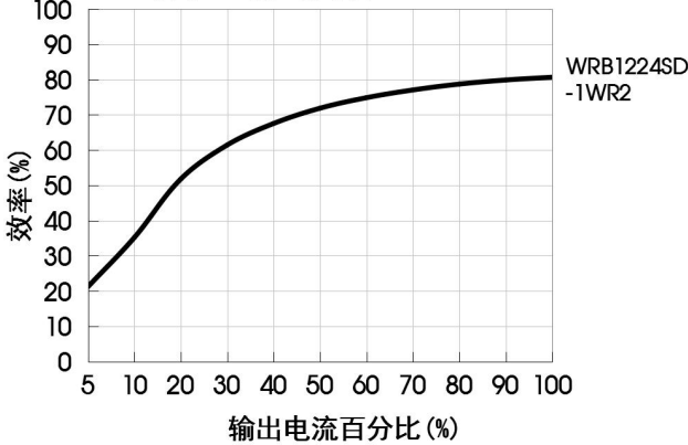
效率Vs输出负载（Vin=12V）
