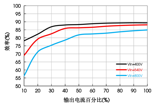
VRF4D28QB-150WR3G-N效率 VS 输出负载
