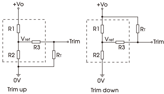
图 5：Trim 使用电路（虚线框为产品内部）
