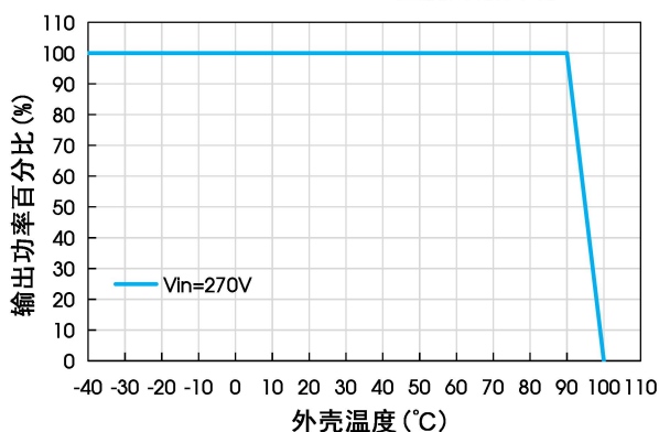
VRF3D05QB-150WR3-N 温度降额曲线
