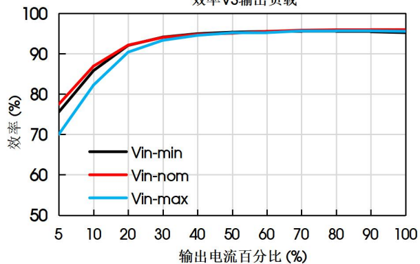
VRF3D48FB-1200WR3 效率VS输出负载
