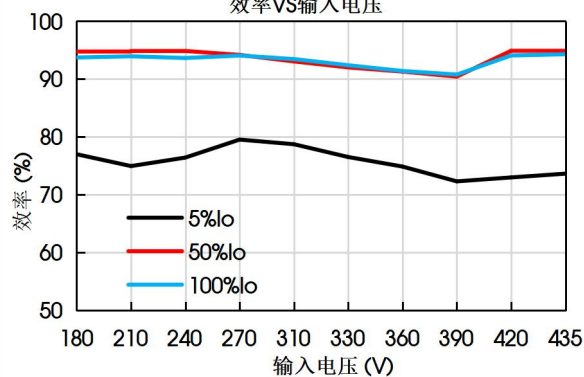
VRF3D24FB-1200WR3 效率VS输入电压
