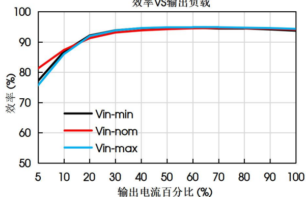
VRF3D24FB-1200WR3 效率VS输出负载
