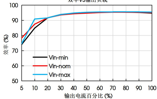
VRF3D48FB-1200WR3 效率VS输出负载
