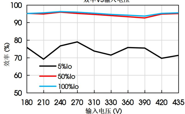
VRF3D48FB-1200WR3 效率VS输入电压
