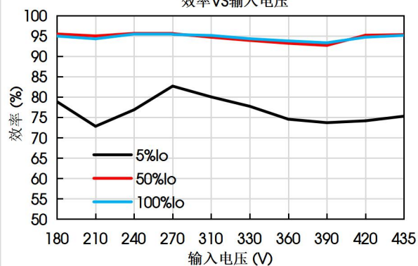
VRF3D28FB-1200WR3 效率VS输入电压
