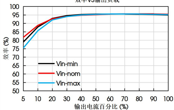
VRF3D28FB-1200WR3 效率VS输出负载
