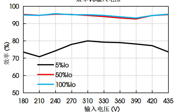
VRF3D48FB-1200WR3 效率VS输入电压
