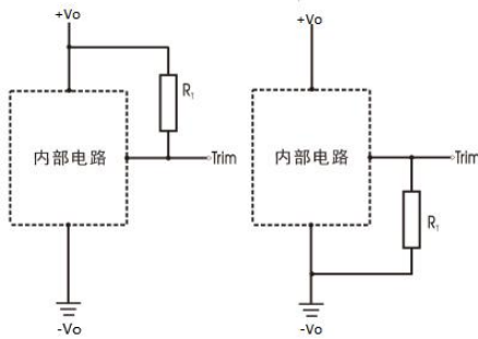
Trim up Trim down 图 5 Trim 的使用电路(虚线框为产品内部)
