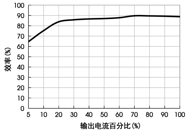
VRB2405SB-75WR3 效率Vs输出负载 (Vin=24V)
