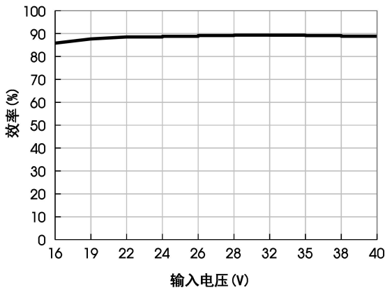
VRB2405SB-75WR3 效率Vs输入电压 (满载)
