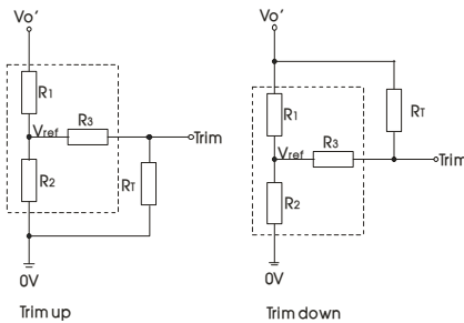
Trim 的使用电路(虚线框为产品内部)：
