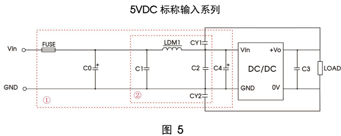
注：图 5 中第①部分用于 EMC 测试；第②部分用于 EMI 滤波，可依据需求选择。
