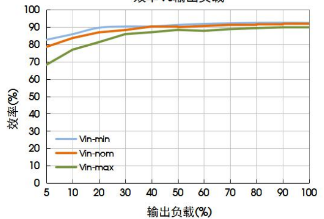
VCF4815SBO-200W(F)R3S(-N) 效率Vs输出负载
