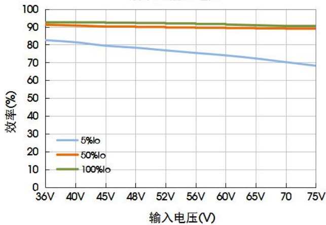
VCF4815SBO-200W(F)R3S(-N) 效率Vs输入电压
