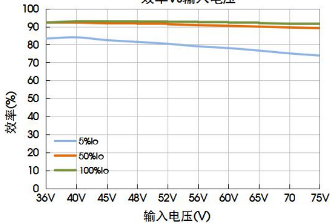
VCF4815SBO-200W(F)R3S(-N) 效率Vs输入电压
