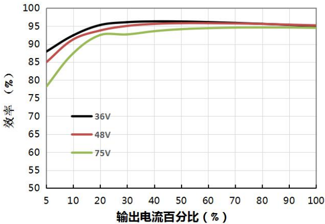
VCF4812QBO-400W(F/H)R3(-N) 效率 VS 输出负载
