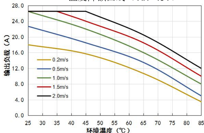
VCF4815QBO-400WR3(-N) 温度降额曲线 (Vin=48V)
