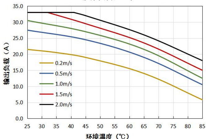
VCF4812QBO-400WR3(-N) 温度降额曲线 (Vin=48V)
