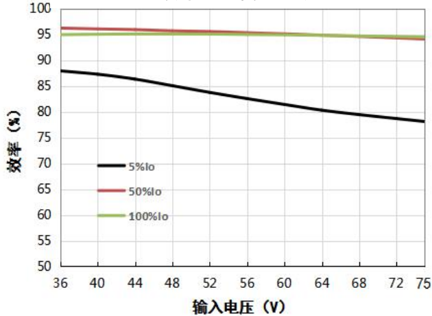
VCF4812QBO-400W(F/H)R3(-N) 效率 VS 输入电压
