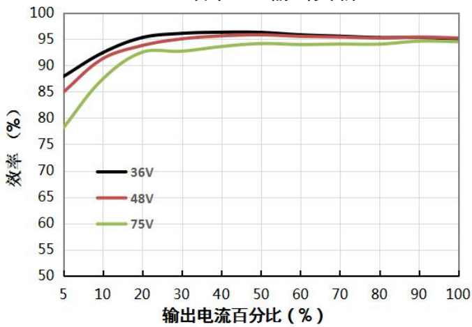
VCF4815QBO-400W(F/H)R3(-N) 效率 VS 输出负载
