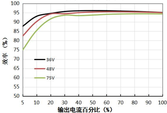
VCF4828QBO-400W(F/H)R3(-N) 效率 VS 输出负载
