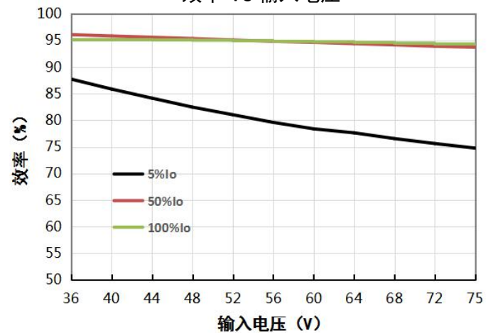
VCF4828QBO-400W(F/H)R3(-N) 效率 VS 输入电压
