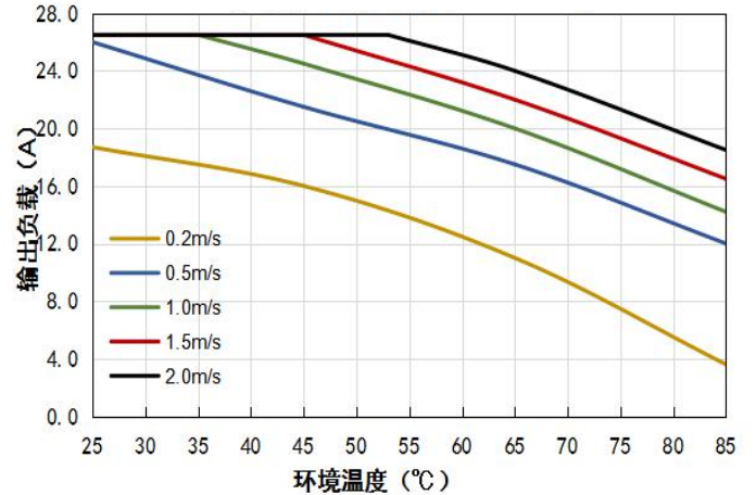
VCF4815QBO-400WFR3(-N) 温度降额曲线 (Vin=48V)
