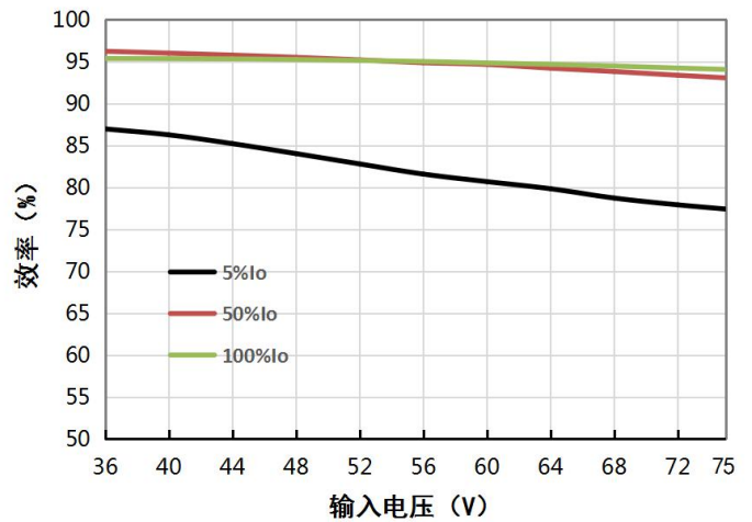
VCF4815QBO-400W(F/H)R3(-N) 效率 VS 输入电压
