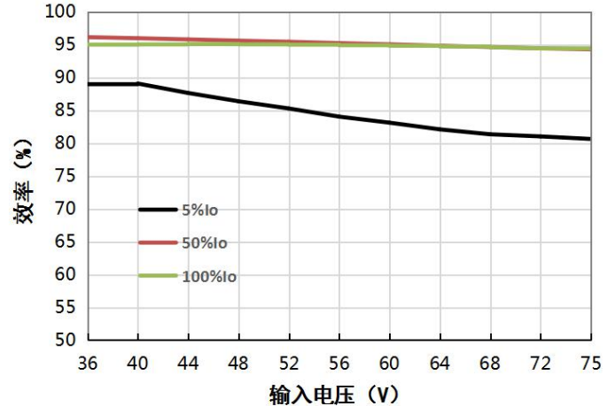
VCF4824QBO-400W(F/H)R3(-N) 效率 VS 输入电压
