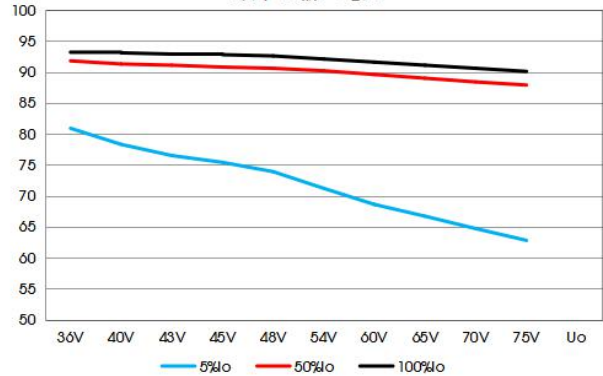
VCF4805EBO-50WR3-N 效率VS输入电压
