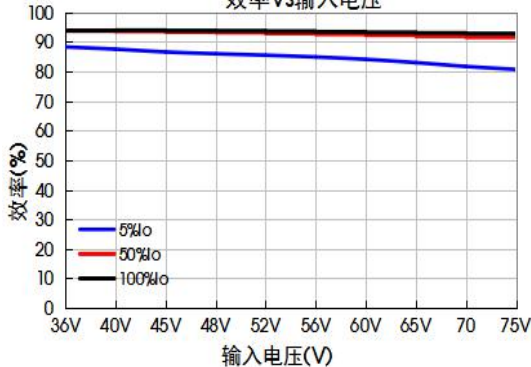
VCF4815EBO-240W(F/H)R3S-N 效率Vs输入电压
