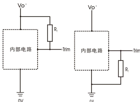
Trim 的使用电路(虚线框为产品内部) 图 9
