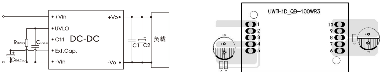
图 7 掉电保持时间推荐电路和 PCB 布局
