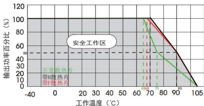
UWTH1D03/05/12/15LD-20W(H/F)R3 温度降额曲线 (Vin=110V, 无风)
