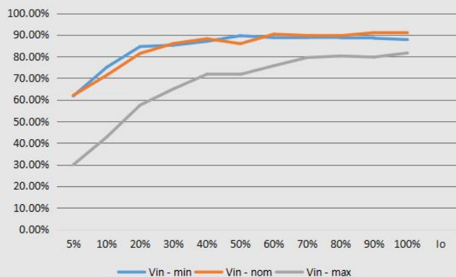
效率随输出负载变化曲线 (常温)
