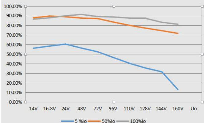
效率随输入电压变化曲线 (常温)
