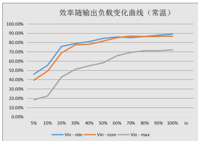
UWTH1D54LD-10WR3 效率随输出负载变化曲线（常温）
