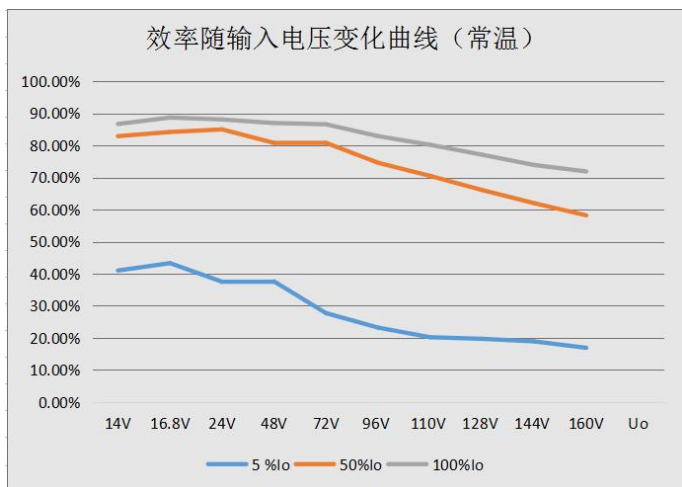
UWTH1D54LD-10WR3 效率随输入电压变化曲线（常温）
