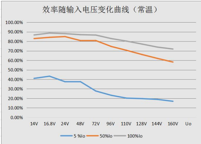
UWTH1D54LD-10WR3 效率随输入电压变化曲线 (常温)
