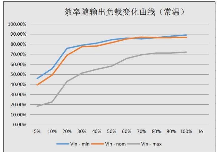
UWTH1D54LD-10WR3 效率随输出负载变化曲线 (常温)
