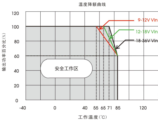
URH2405LP-20WR3 温度降额曲线
