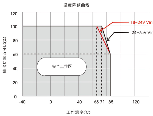
URH4805LP-20WR3 温度降额曲线
