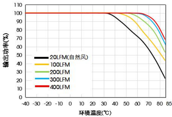
URF4824QB-150WFR3 温度降额曲线 (Vin=24V)
