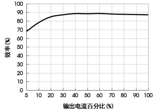
URF1D24QB-50WR3 效率Vs输出负载 (Vin=110V)
