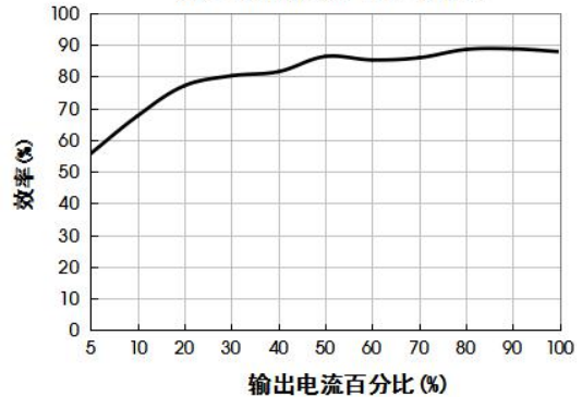
URF1D24QB-50WR3 效率Vs输出负载 (Vin=110V)
