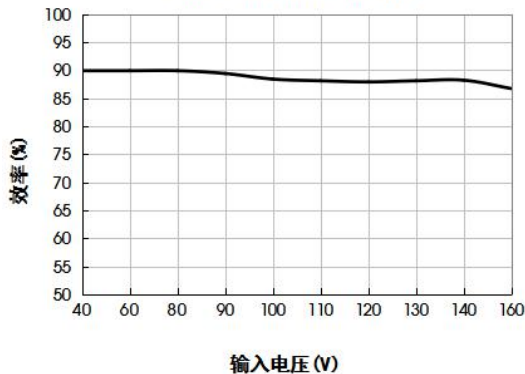
URF1D24QB-50WR3 效率Vs输入电压 (满载)
