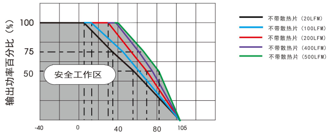
URF1D05QB-100WR3 温度降额曲线 (Vin=110V)
