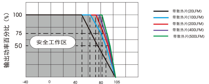
URF1D12QB-100WHR3 温度降额曲线 (Vin=110V)
