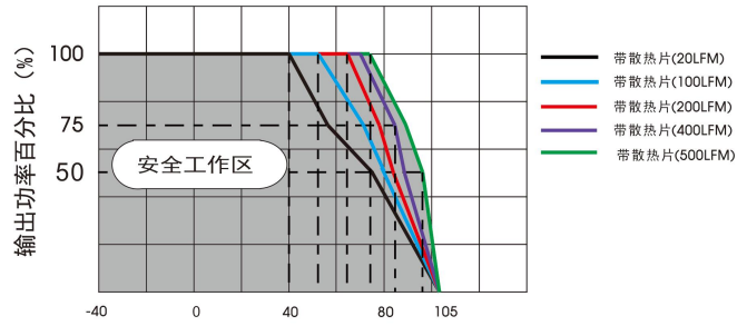
URF1D05QB-100WHR3 温度降额曲线 (Vin=110V)
