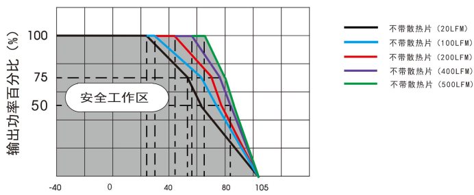
URF1D12QB-100WR3 温度降额曲线 (Vin=110V)
