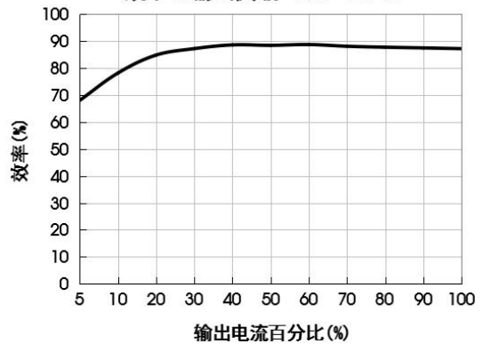
URF1D24QB-100WR3 效率Vs输出负载 (Vin=110V)
