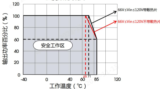
URF1D05LMD-20W(H)R3G 工作温度曲线
