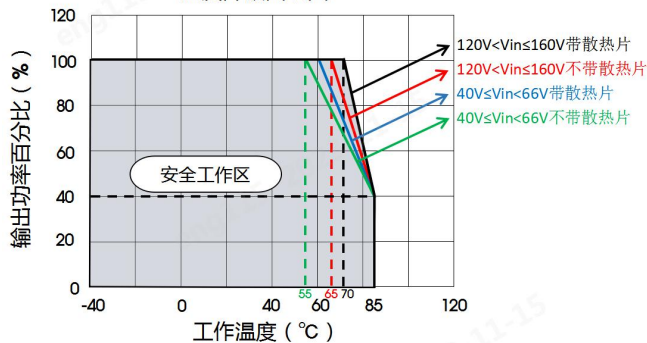
URF1D05LMD-20W(H)R3G 工作温度曲线
