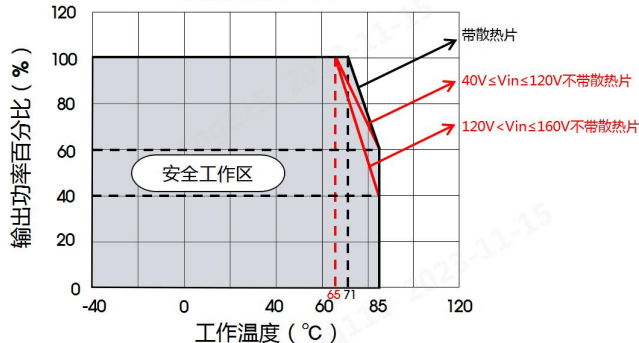
URF1D03LMD-20W(H)R3G 工作温度曲线
