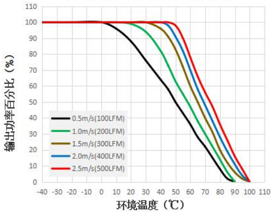
URF1D54FB-400WR3温度降额曲线
