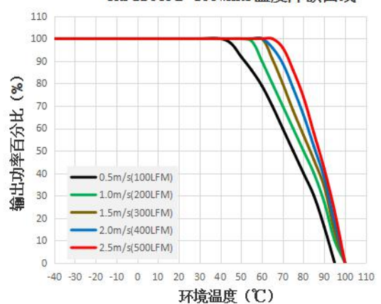
URF1D09FB-400WHR3温度降额曲线
