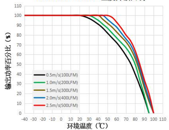
URF1D09FB-400WHR3温度降额曲线
