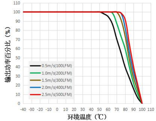
URF1D15FB-400WHR3温度降额曲线
