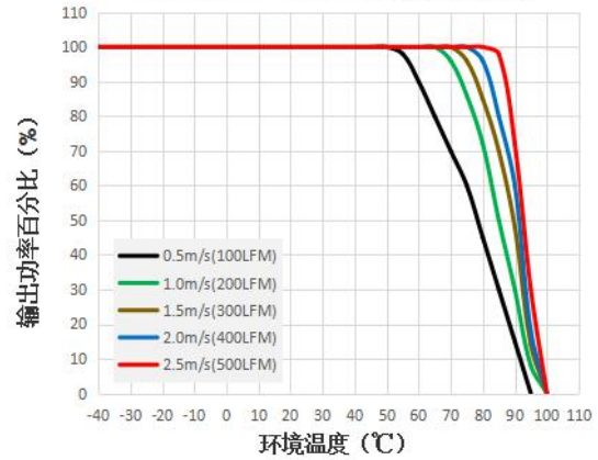
URF1D54FB-400WHR3温度降额曲线
