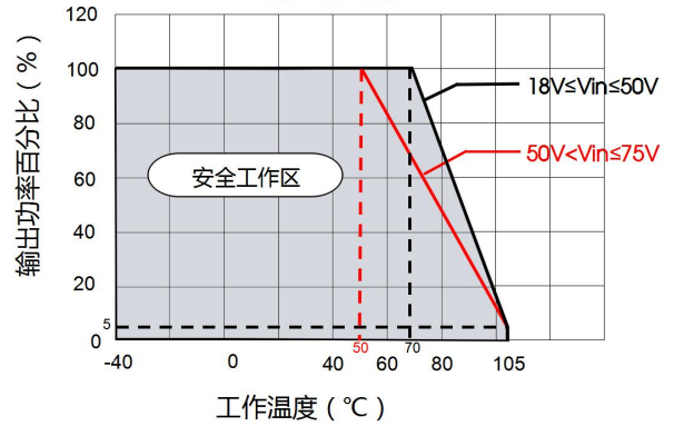
URB4805YMD-40WR3 温度降额曲线图
