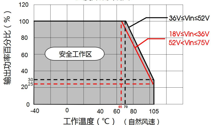
URB4812/15LD-60WHR3 温度降额曲线图
