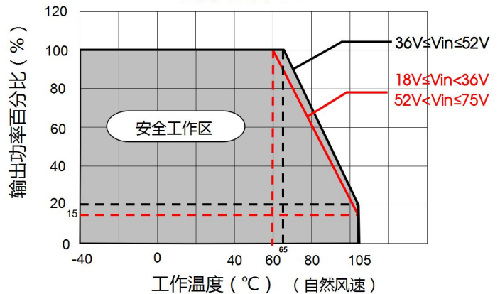
URB4805LD-60WHR3 温度降额曲线图
