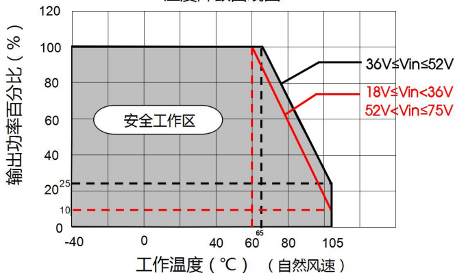
URB4812/15LD-60WR3 温度降额曲线图
