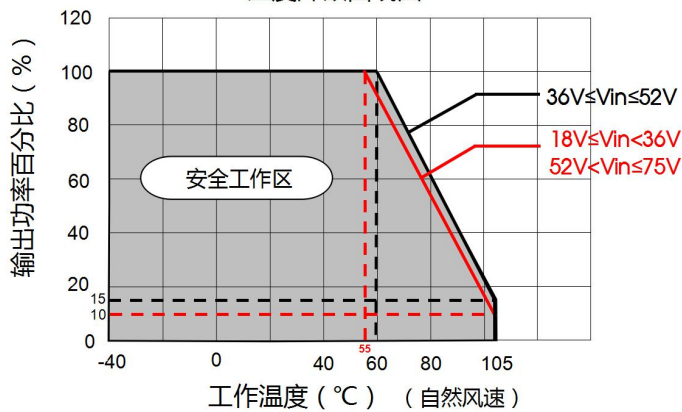
URB4805LD-60WR3 温度降额曲线图
