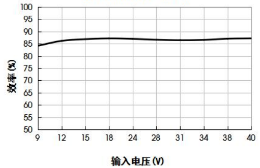
URB2405LN-15WR3G 效率Vs输入电压 (满载)
