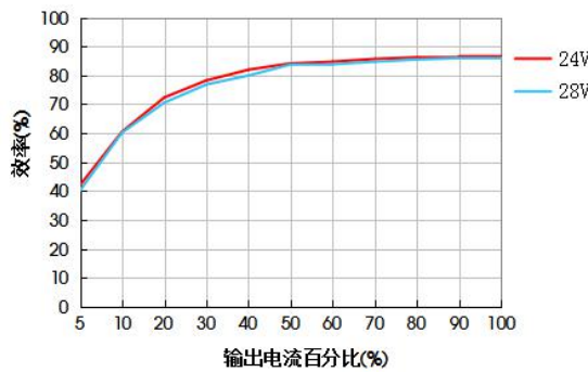
URB2405LN-15WR3G效率Vs输出负载
