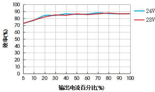
URB2412LN-15WR3G效率Vs输出负载
