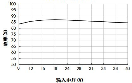
URB2405LN-15WR3G 效率Vs输入电压 (满载)
