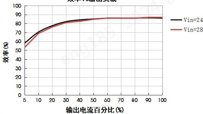
URB2424LN-10WR3G 效率Vs输出负载
