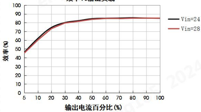
URB2403LN-10WR3G 效率Vs输出负载
