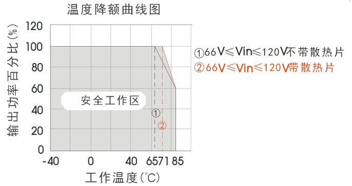
URB1D05LMD-20W(H)R3 工作温度曲线
