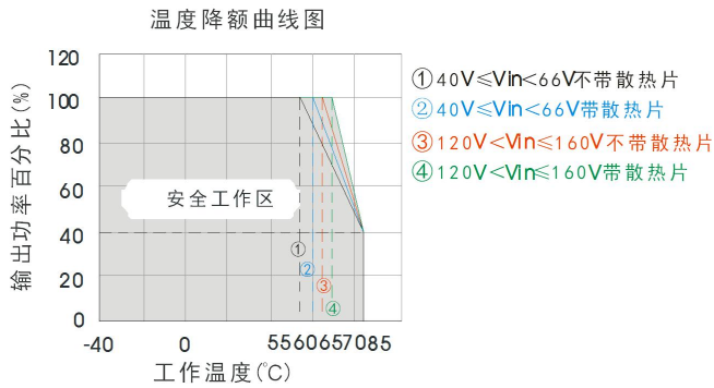
URB1D05LMD-20W(H)R3 工作温度曲线
