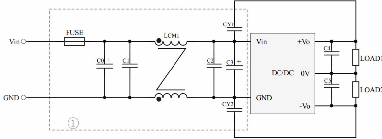
图 4 注: 图 4 中第①部分用于 EMC、EMI 测试;
