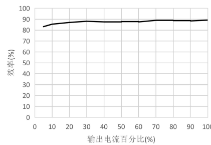
效率Vs输出负载 Vin=24V
