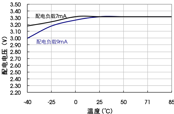
配电电压VS 温度 (T797HL)
