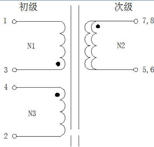
原理图
