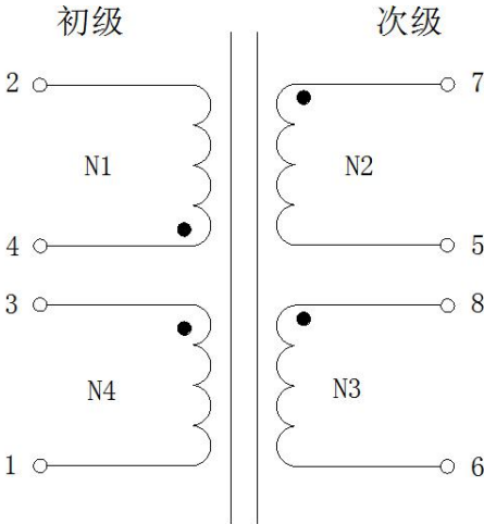
原理图 ● 代表起始点和相位点
