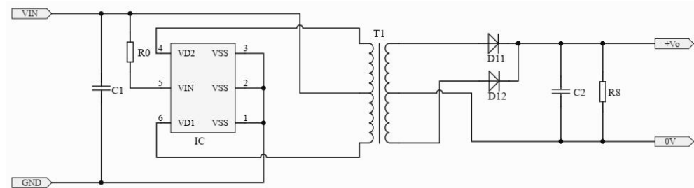
图 3 TTF0503/05/09-1T/2T 应用电路
