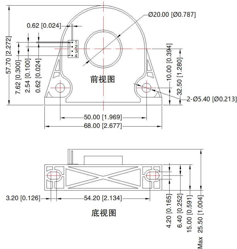
TLx00P-D1C 外观尺寸图
