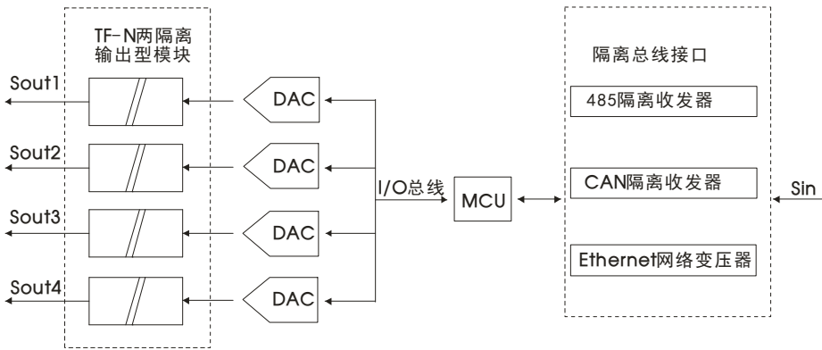
图 3 DCS 系统 AO 板卡隔离应用示意图
