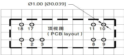
注：栅格距离为2.54*2.54mm
