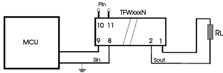
图 2. TFW_N 应用示意图
