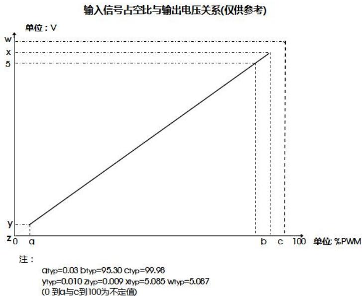
图 4. 输入信号占空比与输出电压关系(仅供参考)
