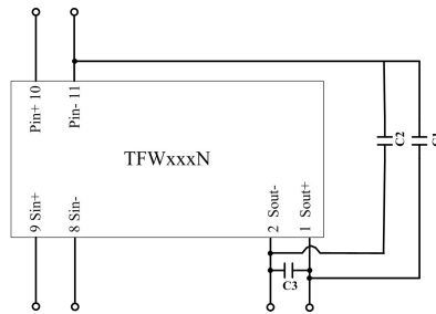
图 3. TFW_N 应用电路推荐外围
