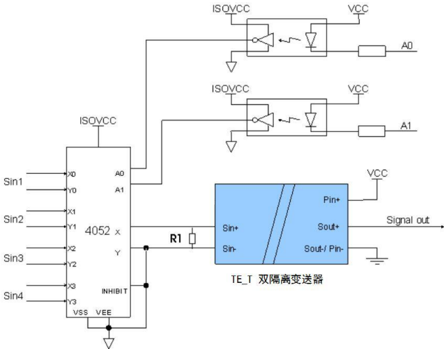
图 3 多通道信号采集应用典型电路
