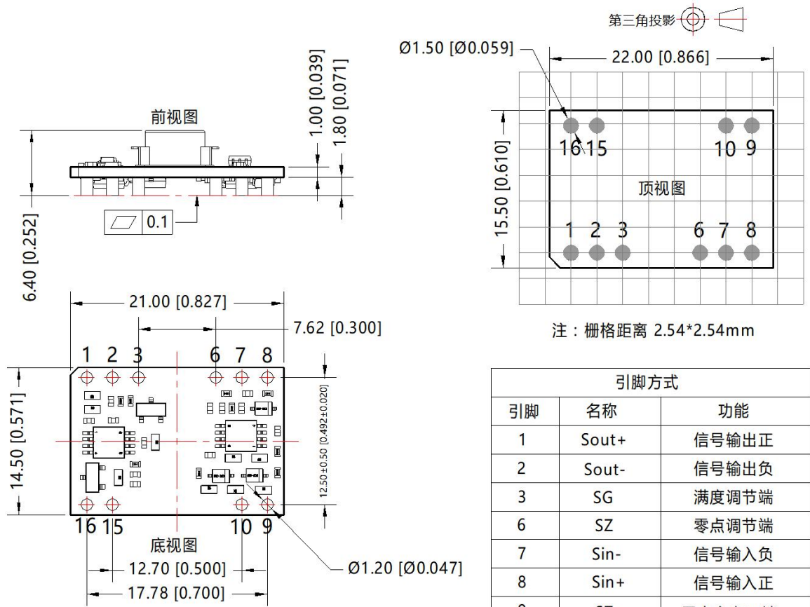
②TE6660T 外观尺寸、建议印刷版图：
