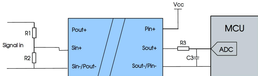
图 4 高电压信号采集应用典型电路
