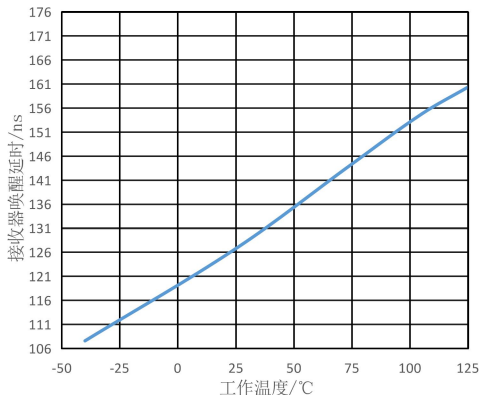
图6.接收器唤醒延时 VS. 工作温度
