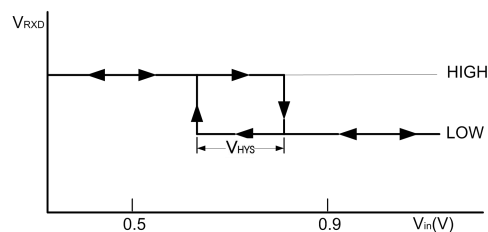
图11.接收回滞电压曲线
