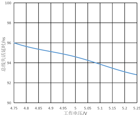
图4.总线失活延时 VS 工作电压
