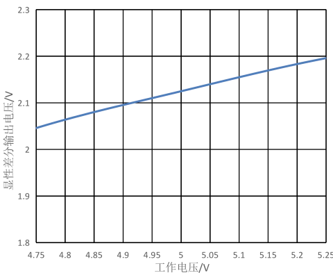
图2.显性差分电压 VS 工作电压
