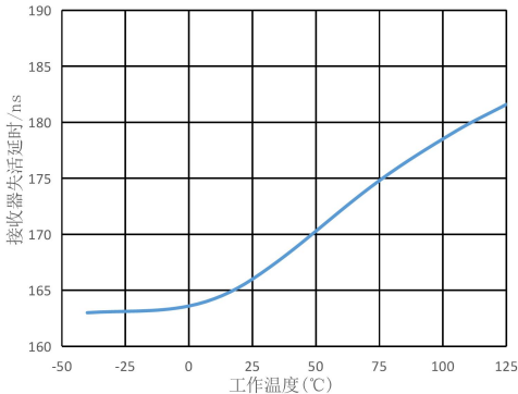
图7.接收器失活延时 vs. 工作温度
