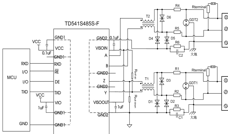
图 13. 端口保护推荐电路
