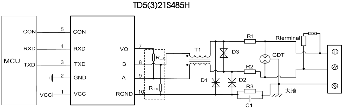
图 2. 端口保护推荐电路
