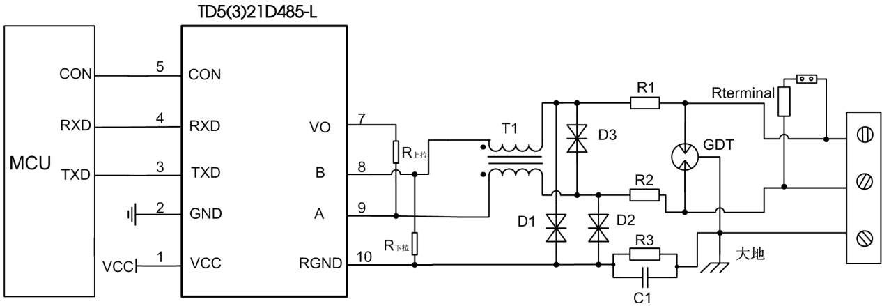
图 2. 推荐防护电路
