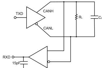
图13.传输特性测试电路
