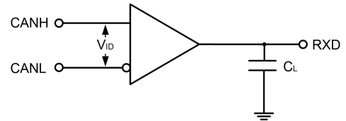
图12.接收器测试电路
