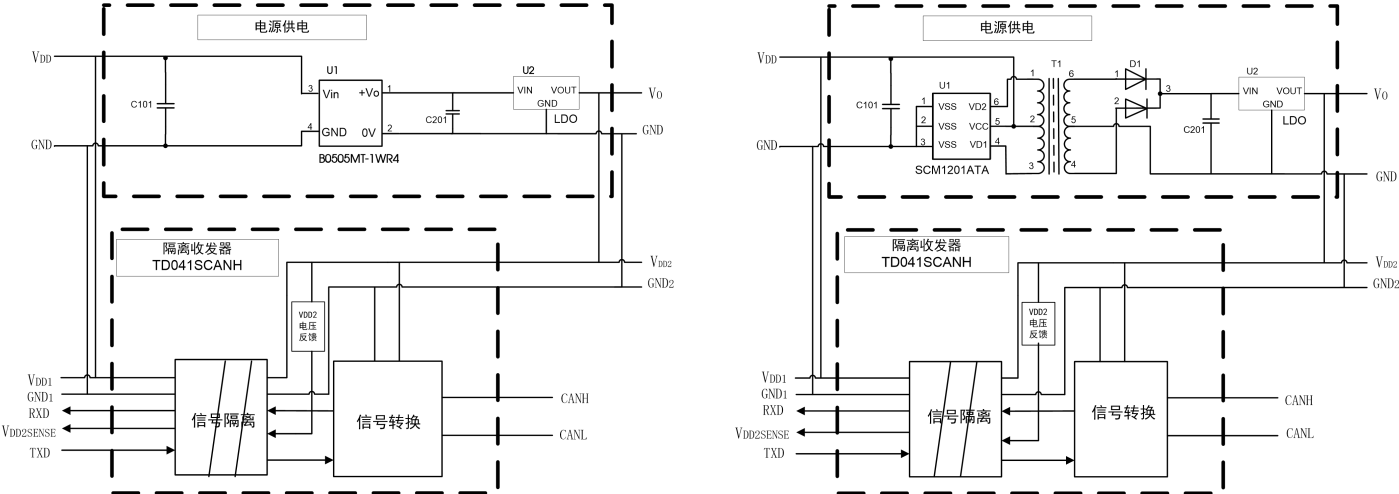
图 16.典型应用电路
