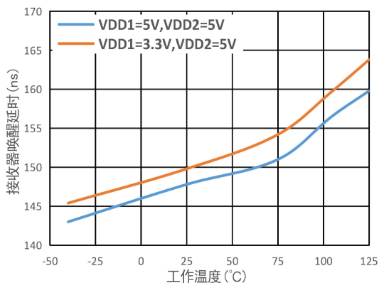
图3. 接收器唤醒延时 vs. 工作温度
