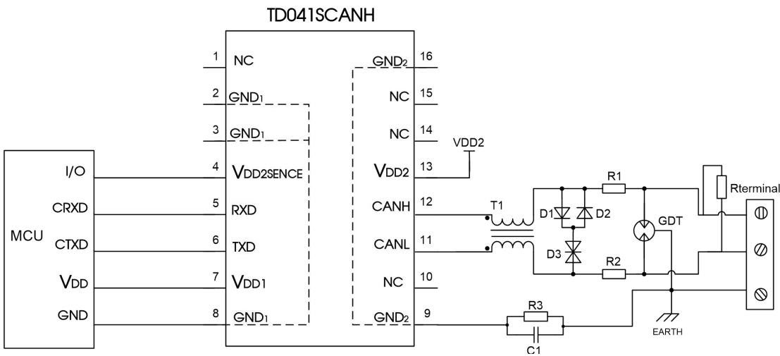
图 17.端口保护推荐电路
