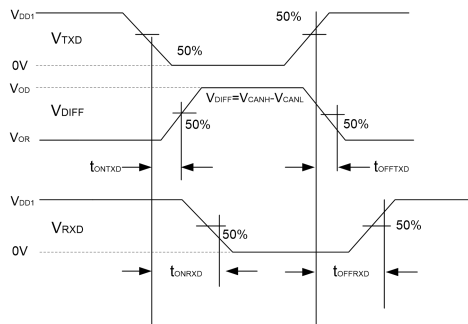
图15.驱动器/接收器传输延时
