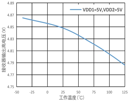
图9.接收器输出高电压 vs. 工作温度
