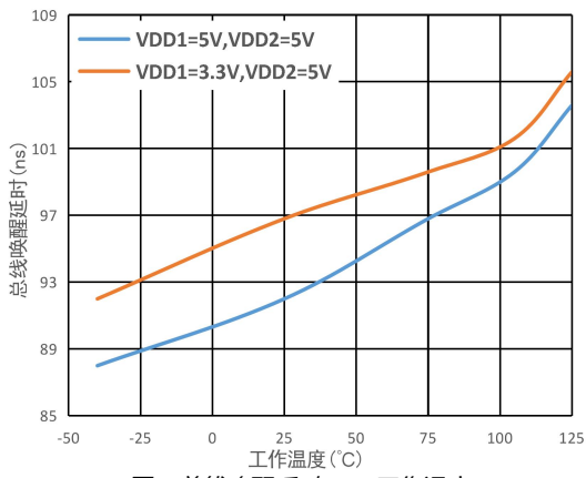
图7.总线唤醒延时 vs. 工作温度
