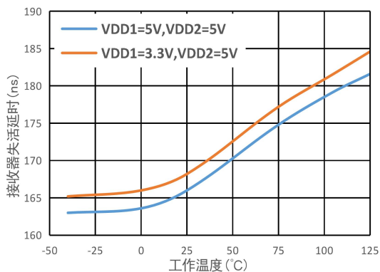
图5. 接收器失活延时 vs. 工作温度
