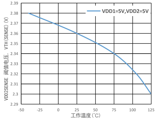
图10.VDD2 反馈电压阈值 vs. 工作温度
