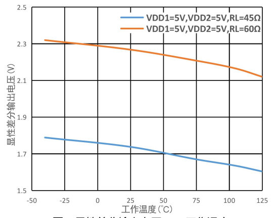
图8.显性差分输出电压 vs. 工作温度
