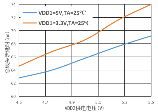
图6. 总线失活延时 vs. VDD2 供电电压
