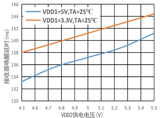
图4. 接收器唤醒延时 vs. VDD2 供电电压
