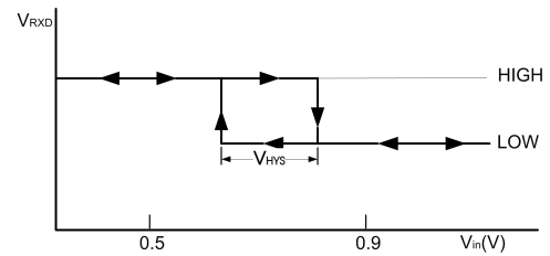
图12.接收回滞电压曲线
