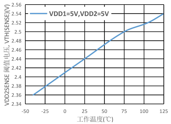
图8.VDD2 反馈电压阈值 vs. 工作温度
