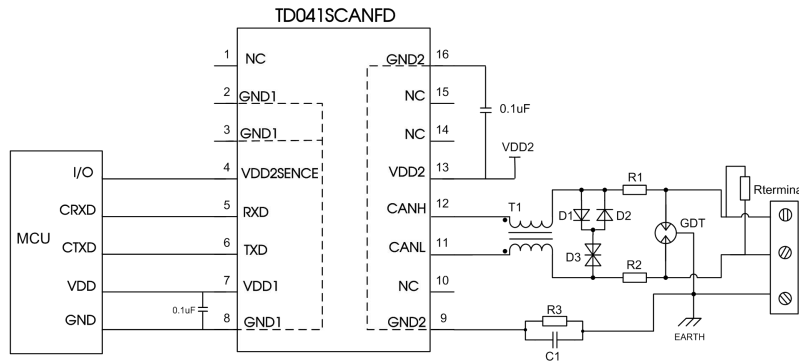
图 15. 端口保护推荐电路
