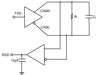
图11.传输特性测试电路
