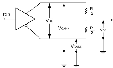
图9.驱动器测试电路
