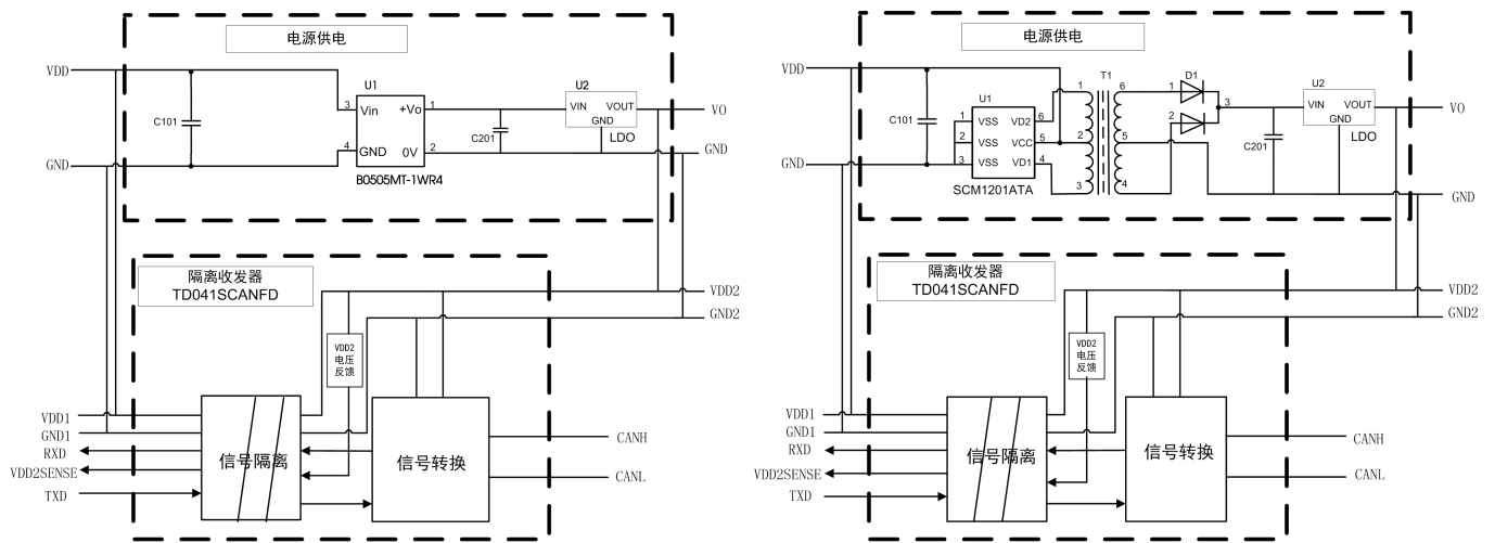
图 14. 典型应用电路
